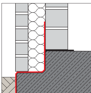
Tætning ved skalmur
