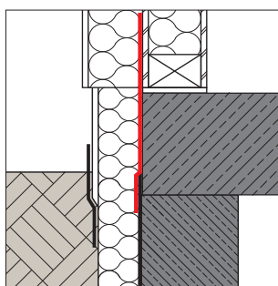
Sokkeltætning ved træbyggeri
