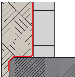
Jordberørte udvendige tætninger
