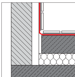
Tætningsmembran under fliser og plader
