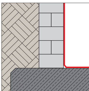
Indvendig tætning af gulv og vægge
