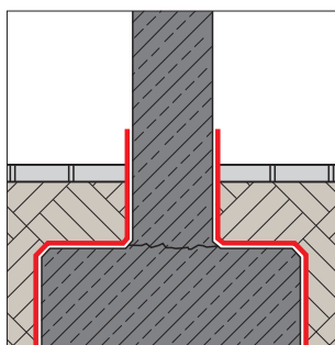
Tætning af søjlefundamenter
