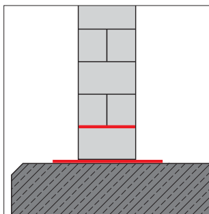
Tætning i og under vægge
