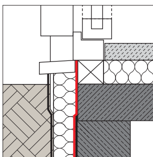
Tætning ved gulv-til-loft vinduer
